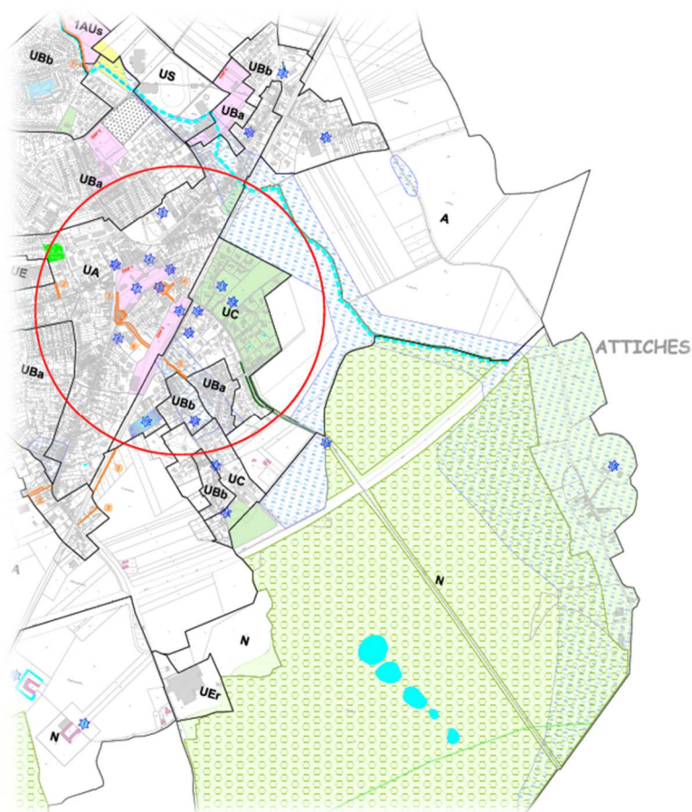
Figure 14 : Identification des limites des secteurs concernés par des zones inondées constatées
